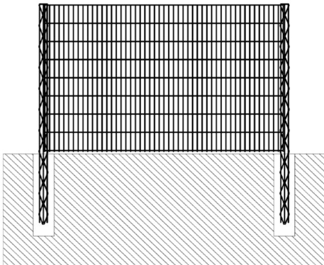
Рис. 2 Установка на грунт
