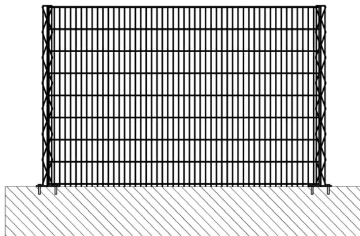
Рис. 3 Установка на твердое основание
